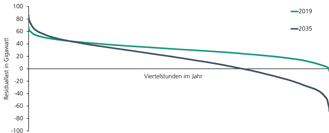
Abbildung 4: Dauerlinien der Residuallast in Deutschland für die Jahre 2019 und 2035. Quellen [8, 9], eigene Darstellung.
