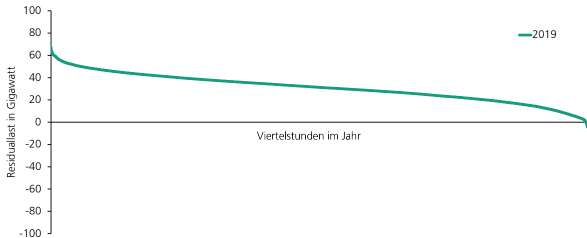
Abbildung 1: Dauerlinie der Residuallast in Deutschland im Jahr 2019. Quelle: [8], eigene Darstellung.
